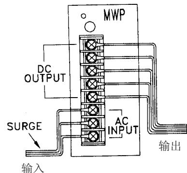
图八 配线及连接
