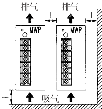
图五 多台使用时需考虑通风距离
