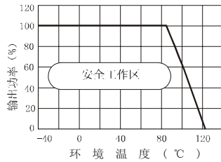
温度曲线图
