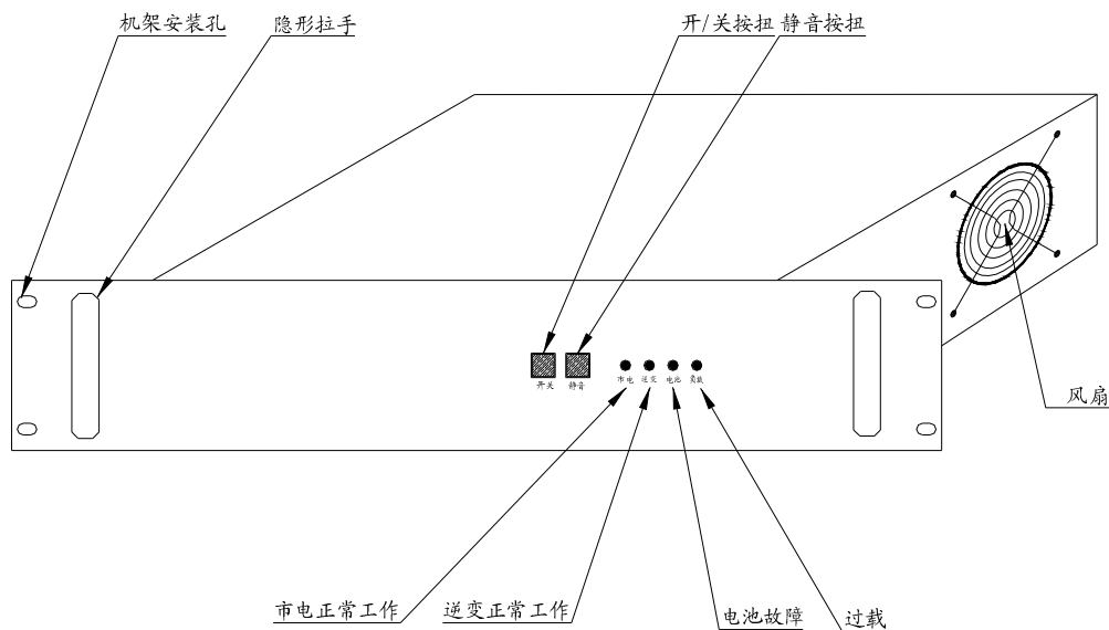
图一：500VA 电源机箱前视图（2U/19 英寸机架式）
