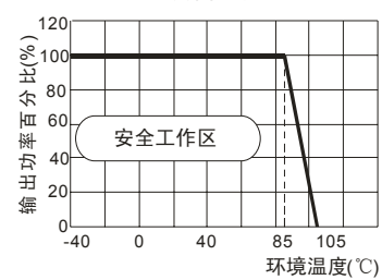
温度曲线图
