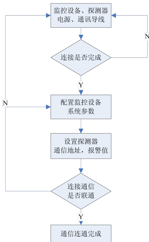
图 3 调试流程图
