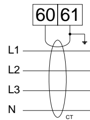
三相四线漏电电流检测
