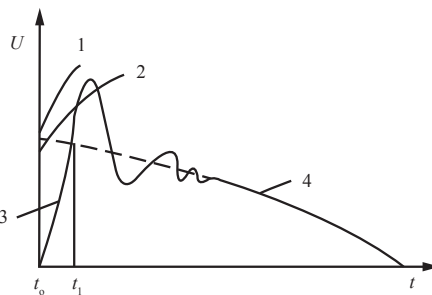
1-- 绝缘强度恢复高于避雷器恢复电压； 2-- 绝缘强度恢复低于避雷器恢复电压； 3-- 避雷器恢复电压；4-- 工频电压
