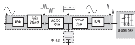
图 2 传统 UPS 系统结构
