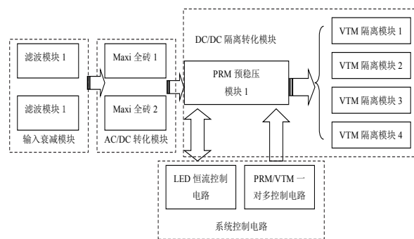
图 1 新型 LED 驱动电源整体原理框图
