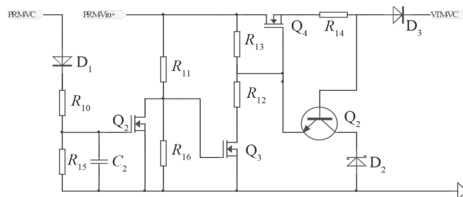
图 2 PRM/VTM 一对多输出控制电路
