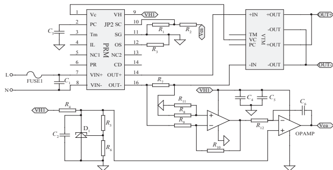
图 3 恒流控制电路图
